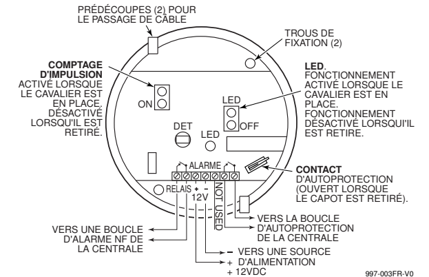
Figure 3. Circuit imprimé du détecteur (placé dans l'embase)
