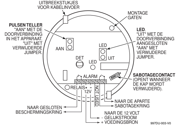
Figuur 3. Printplaat (In de Basis Van de PIR)
