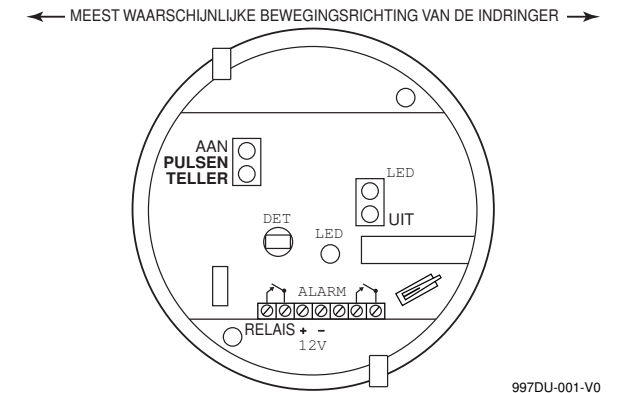
Figuur 1. Optimale Plaats Van Bevestiging
