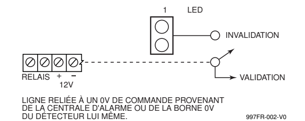
Figure 2. Commande à distance de la LED
