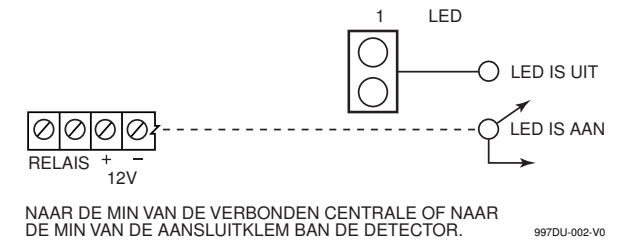
Figuur 2. Bediening Van De LED Op Afstand
